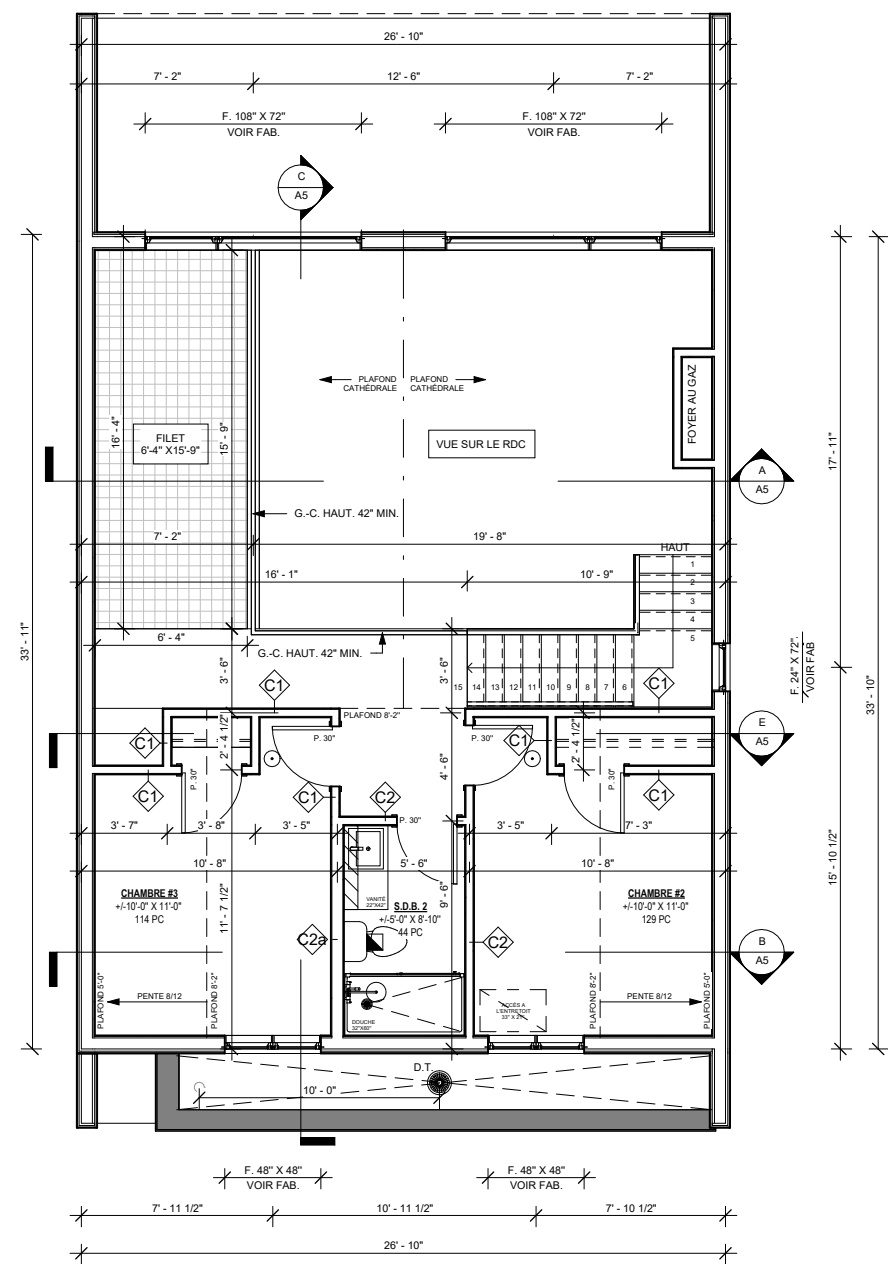
PLAN REZ-DE-CHAUSSÉE + 1
