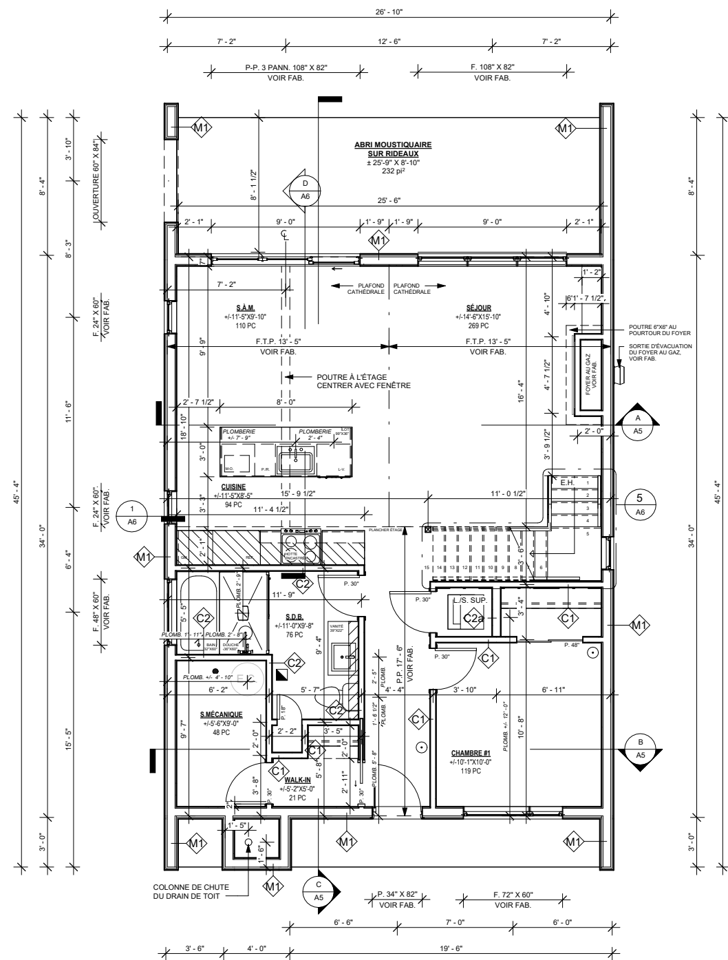
PLAN REZ-DE-CHAUSSÉE
