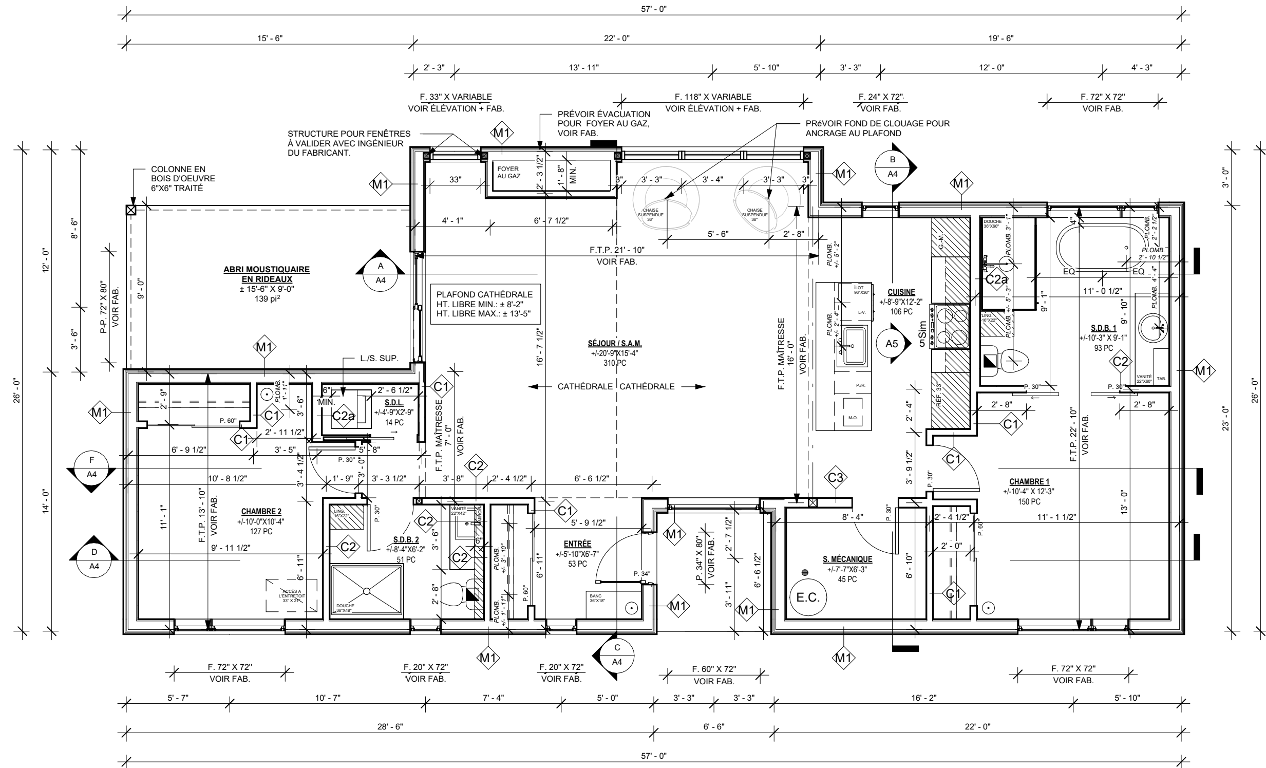
PLAN REZ-DE-CHAUSSÉE
